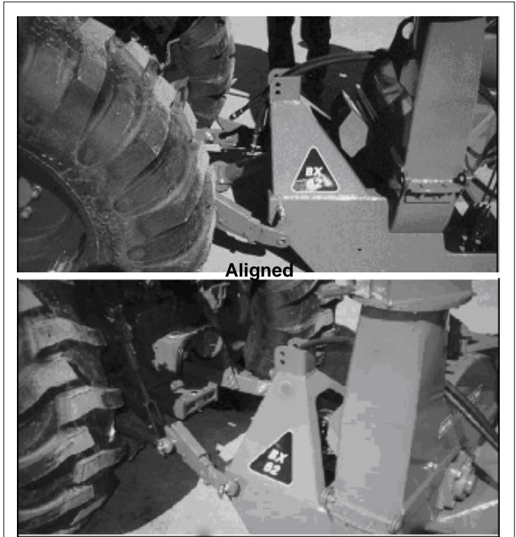
Fig. 15 LOWER ARMS
