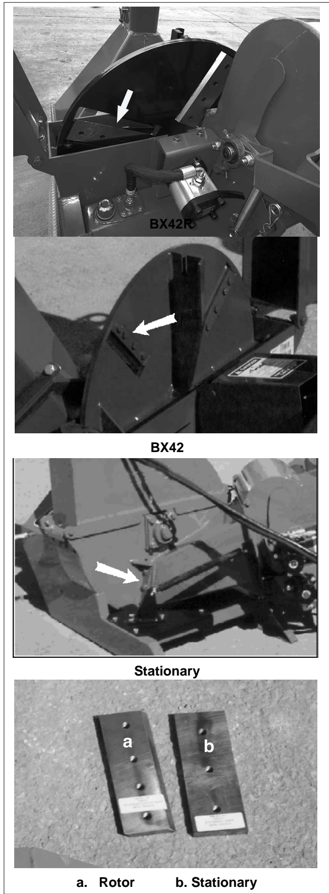
Fig. 32 BLADES
